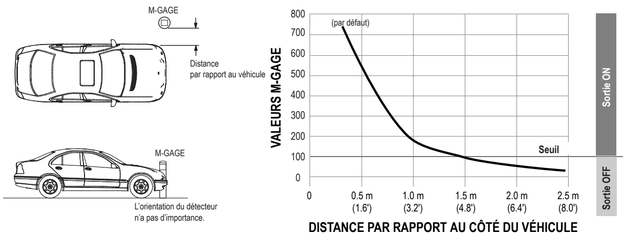
Illustration 3. Lecture des valeurs M-GAGE avec une installation à 1 mètre au-dessus du sol.
