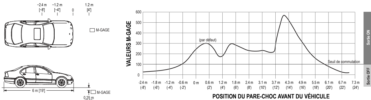
Illustration 4. Lecture des valeurs M-GAGE avec une installation sous terre.
