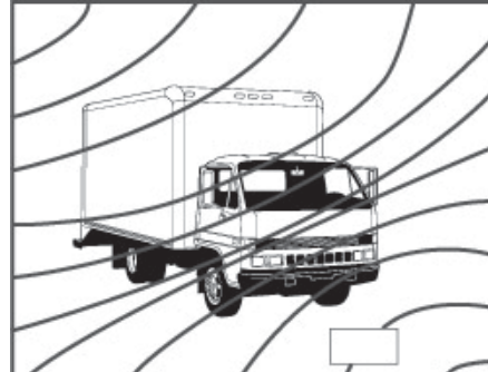
Illustration 2. Champ B : après l'introduction d'un objet de grande taille, le champ magnétique change. Le détecteur perçoit les modifications d'intensité et d'orientation entre le champ ambiant et le champ B. Si la différence est supérieure au seuil de sensibilité, le dispositif signale un changement d'état.
